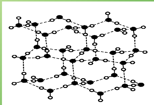
冰的结构
